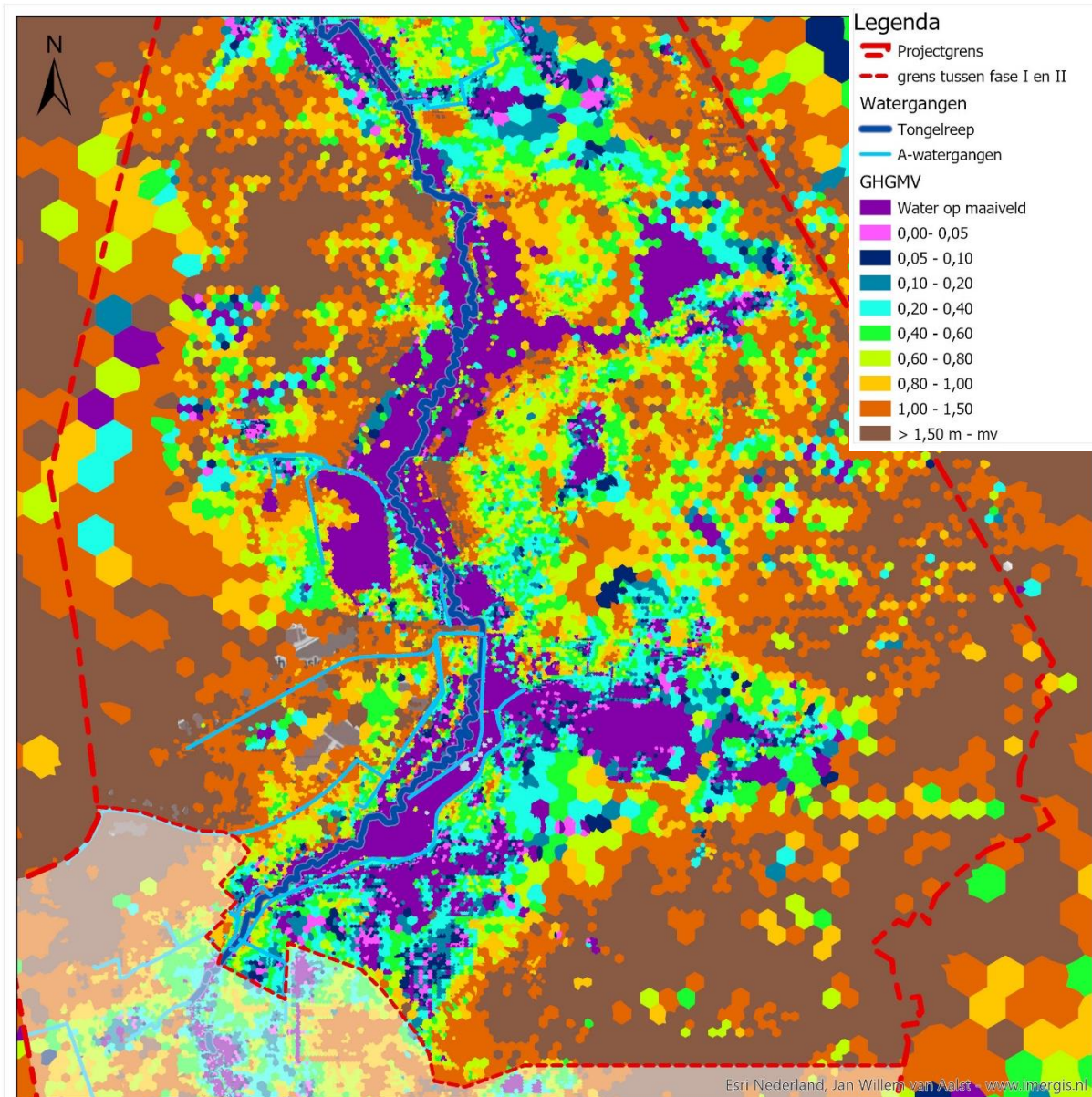
Figuur 1.6-2 B. Gemiddelde Hoogste Grondwaterstand (GHG) VKA t.o.v. mv
