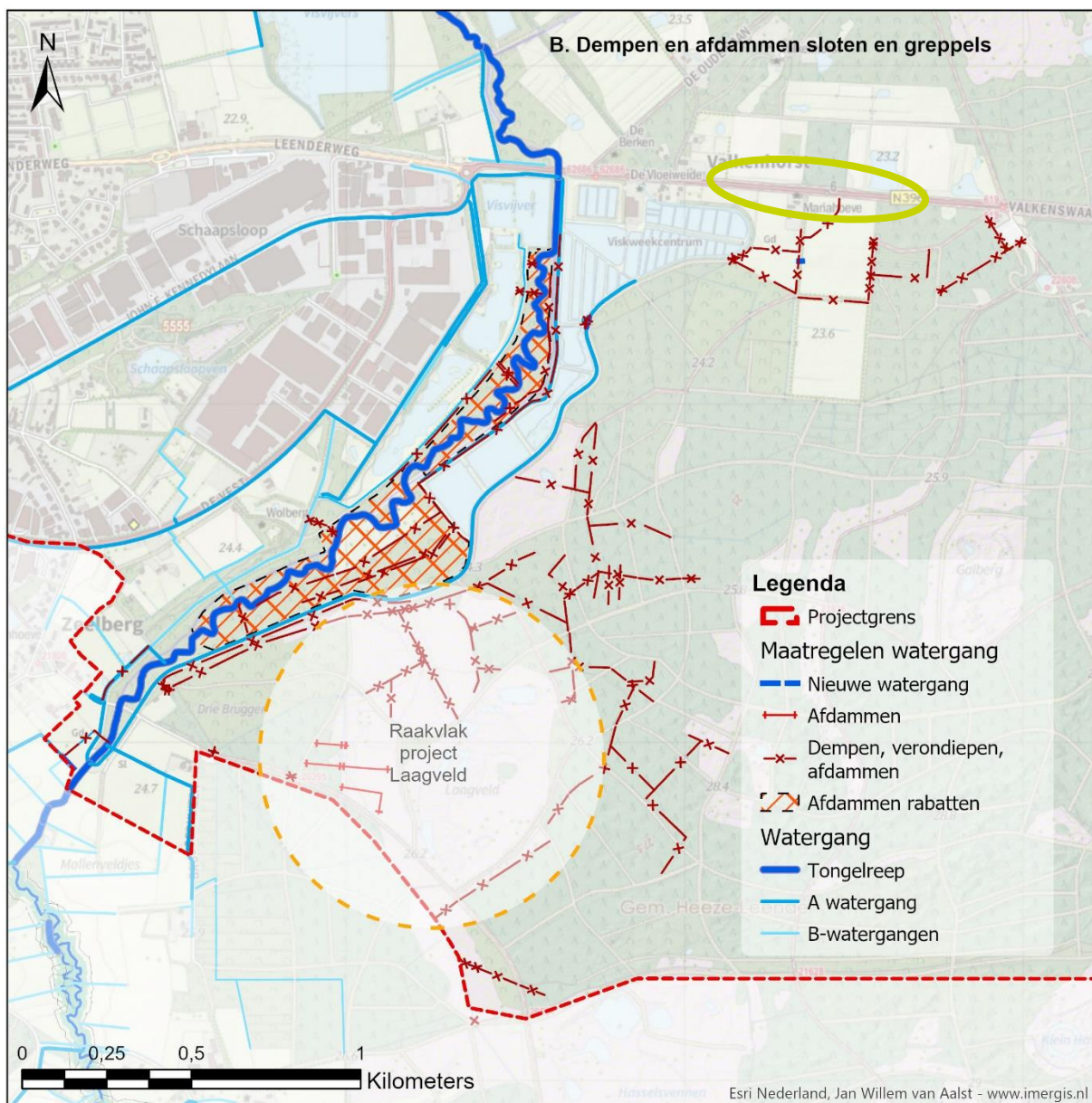
Figuur 1.5-5 Maatregelen m.b.t. dempen, afdammen en verondiepen greppels en sloten
