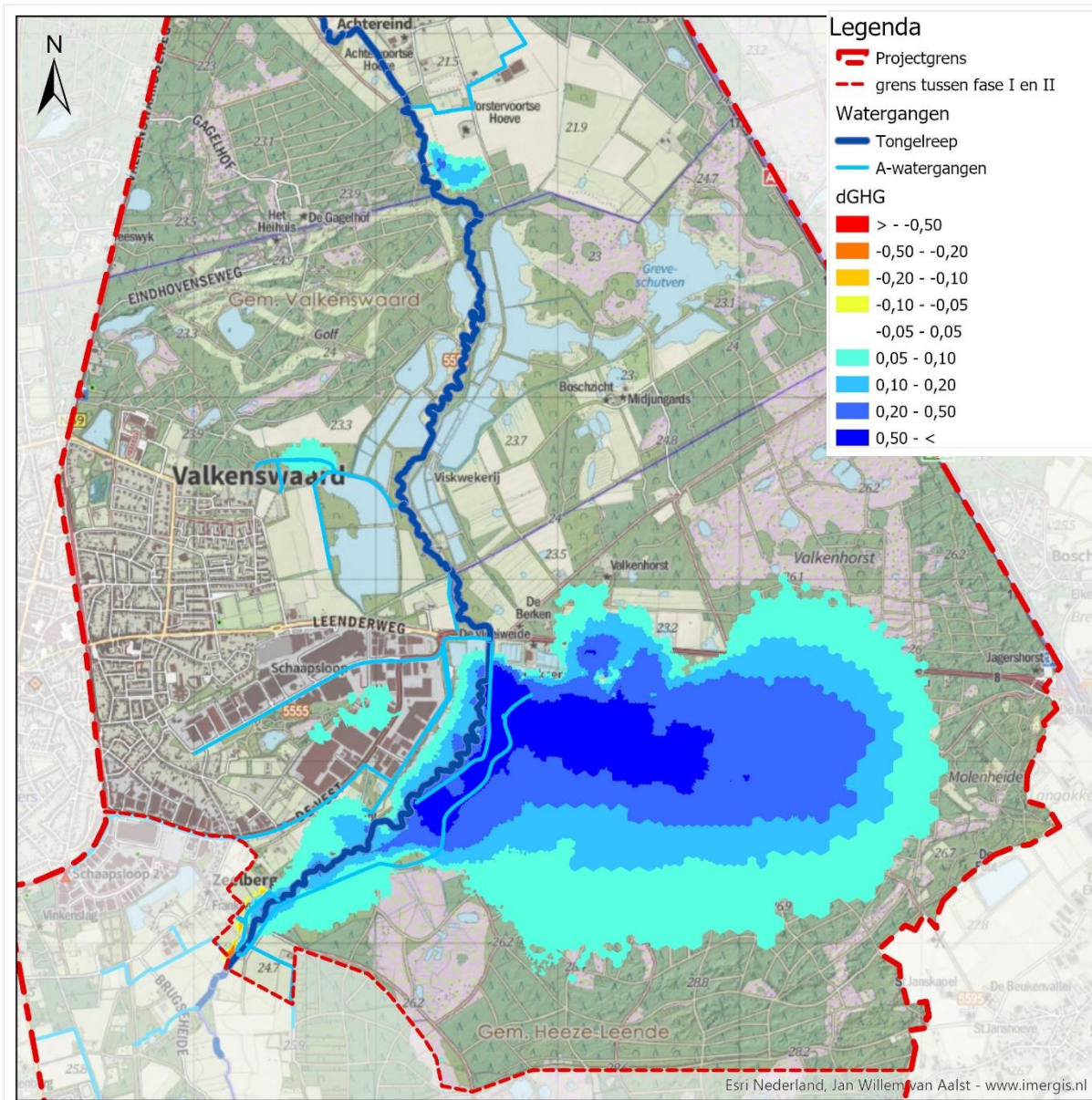
Figuur 1.6-1 A. Verandering GHG t.o.v. referentie
