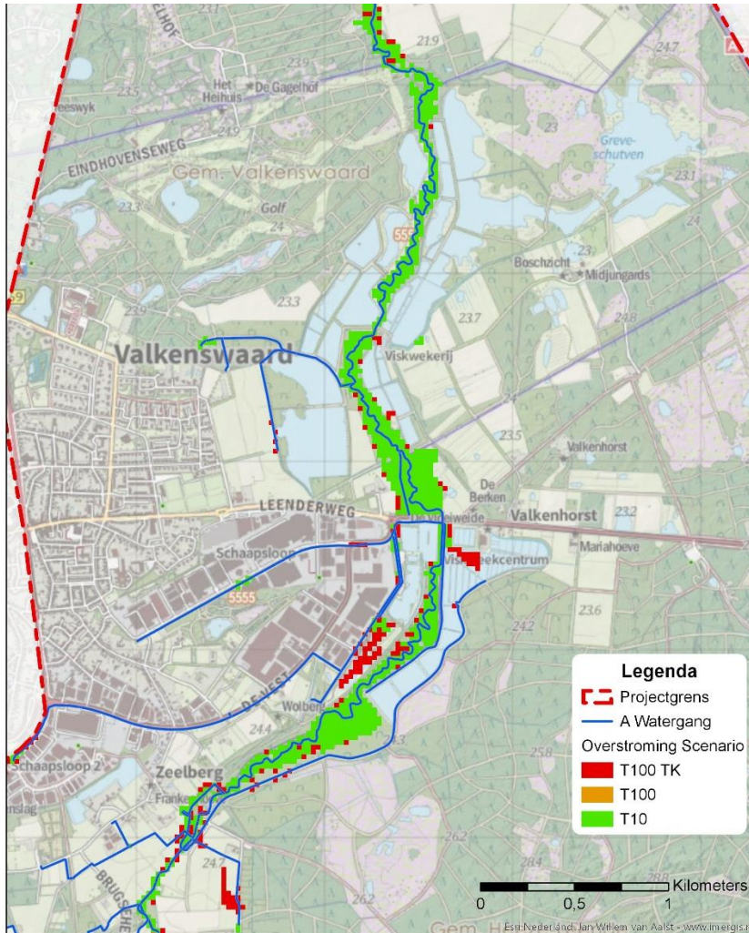
Figuur 1.6-5 Overstromingsbeelden bij de Tongelreep Scenario
